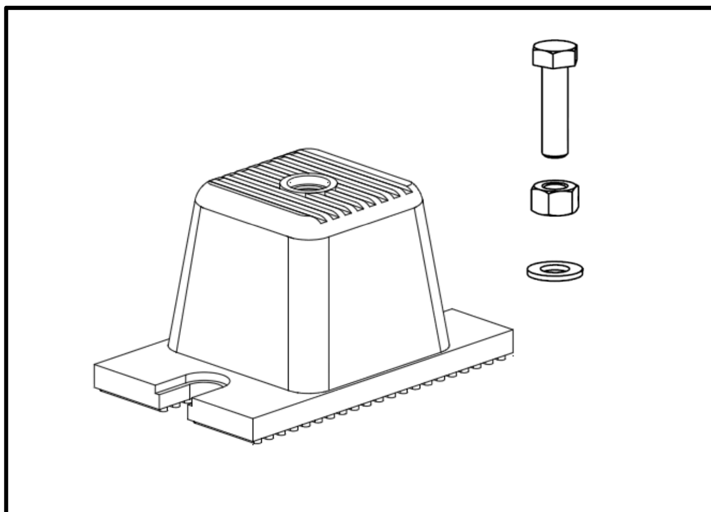
圖1)檢查附件是否齊全，避震器有無缺陷破損。
