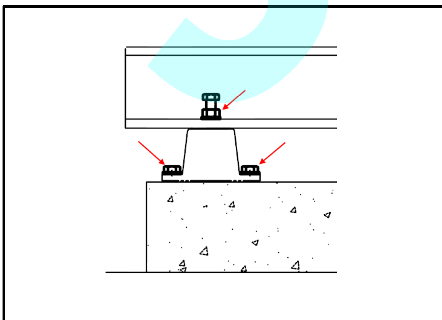
圖3)鎖緊螺母和墊圈，確保設備和避震器固定。
