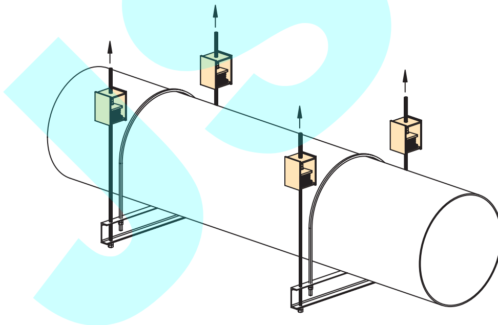
安裝示意圖 Installation illustration
