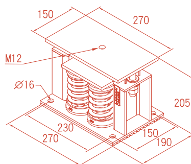
JA-4-B 配件
