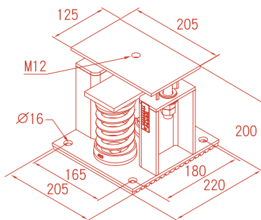
JA-2-B 配件
