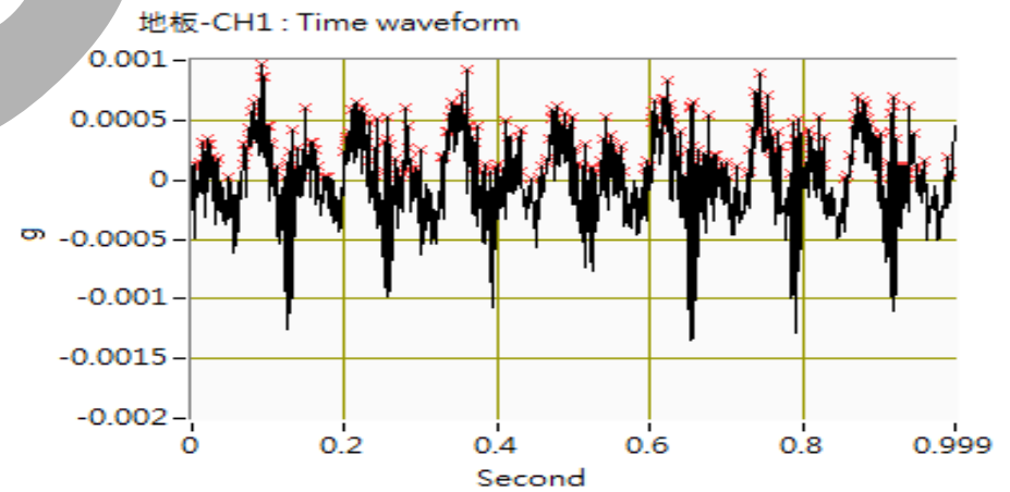
裝設氣墊式避震器-地面端震動數據
