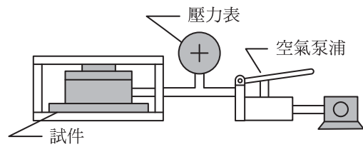
氣墊式避震器 橡膠耐壓試驗系統圖
